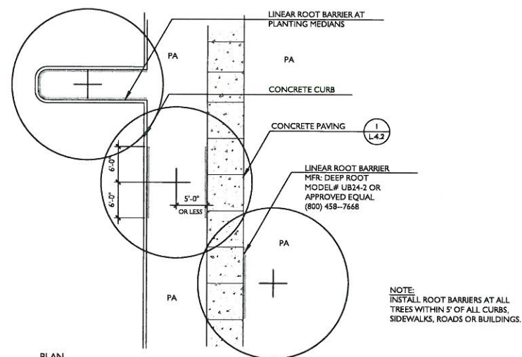
2 LINEAR ROOT BARRIER SCALE: 1" = 10'-0"
