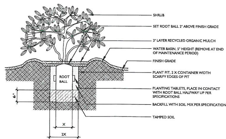
4 SHRUB PLANTING SCALE: N.T.S.
